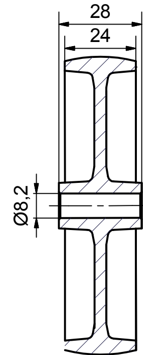
SECTION A-A'
